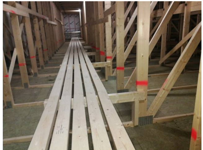
Ullakolla 500 mm korkomerkki, korot maalattu villan puhalluksen vahvuuden seuranta varten.
